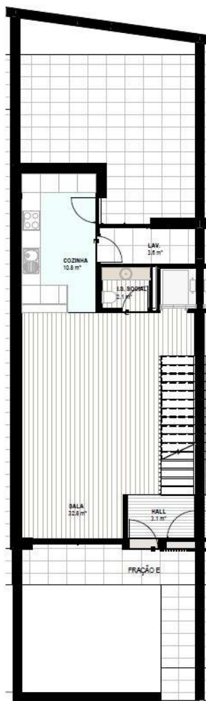
E - Piso 0
